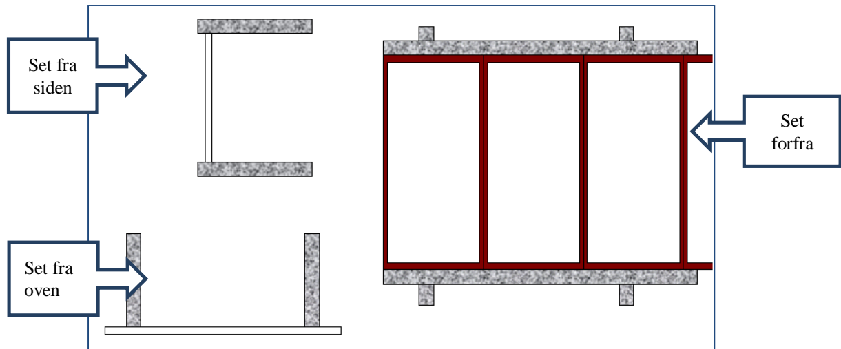
Figur 3: Vandret vinduesbånd
